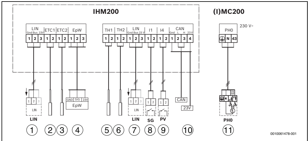
Bild 3 Überblick Anschlussklemmenbelegung
