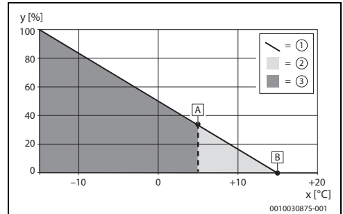
Afb. 2 Buitentemperatuur alternatief
