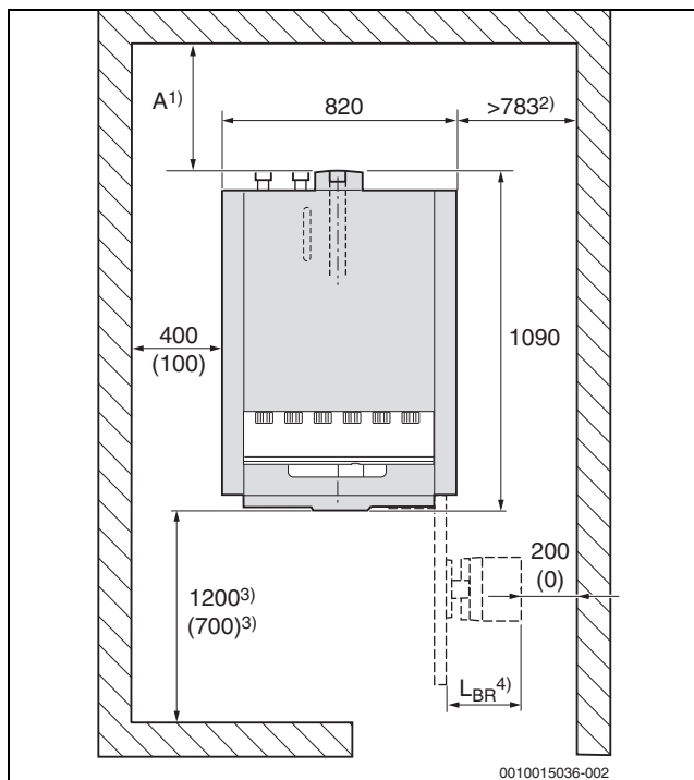
Bild 7 Aufstellraum Maße in mm → Tabelle 10, Seite 18 (Werte in Klammern sind Mindestabstände)
