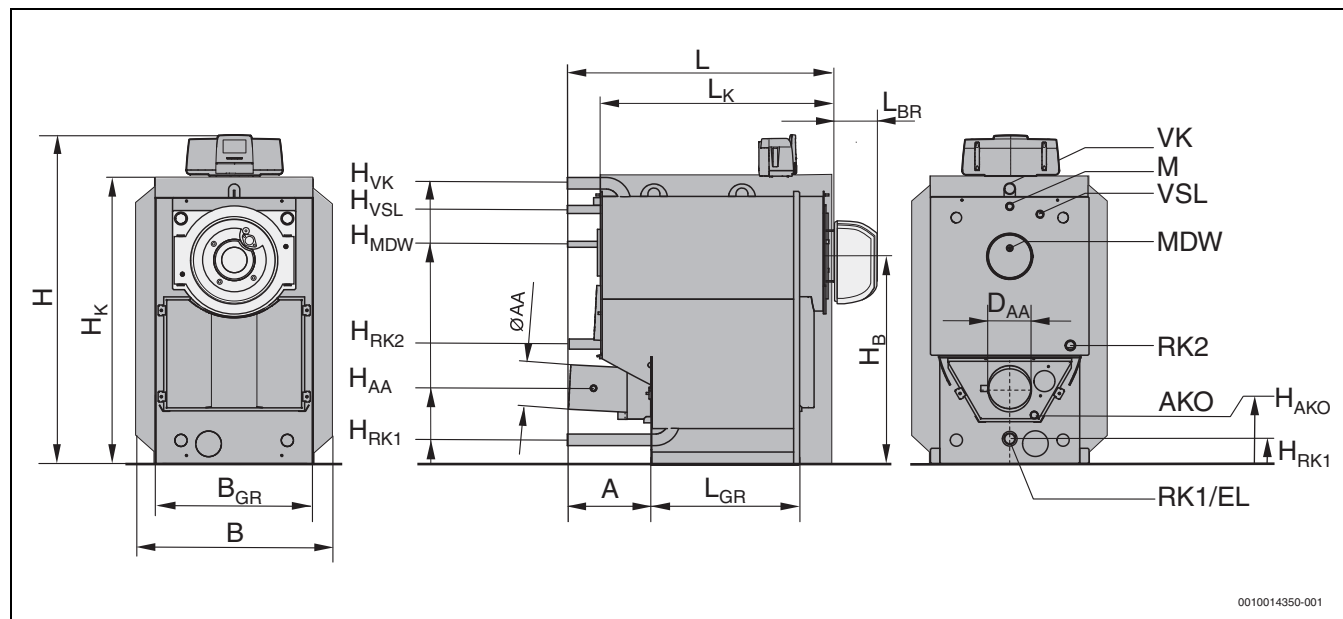
Bild 3 Anschlüsse und Abmessungen
