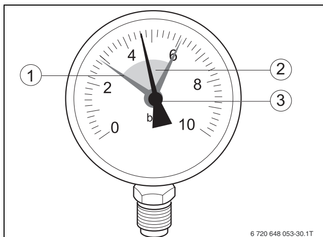
Bild 45 Manometer für geschlossene Heizungsanlagen
