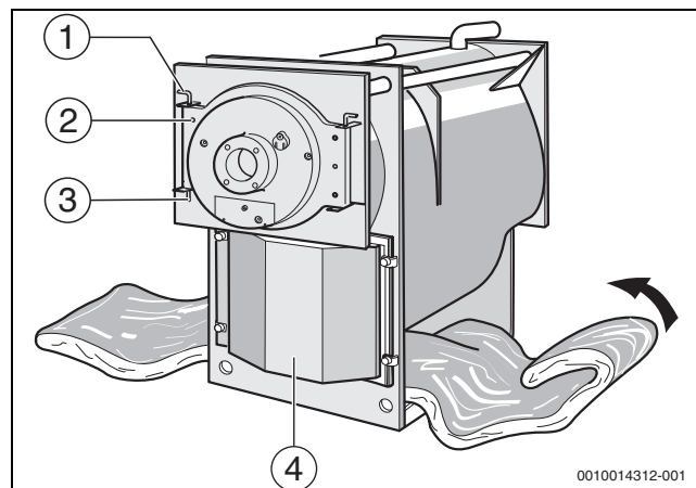
Bild 9 Wärmeschutzmatte unter dem Kessel durchschieben
