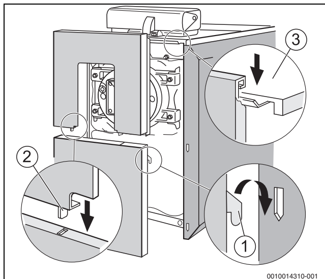
Bild 22 Obere und untere Vorderwand befestigen
