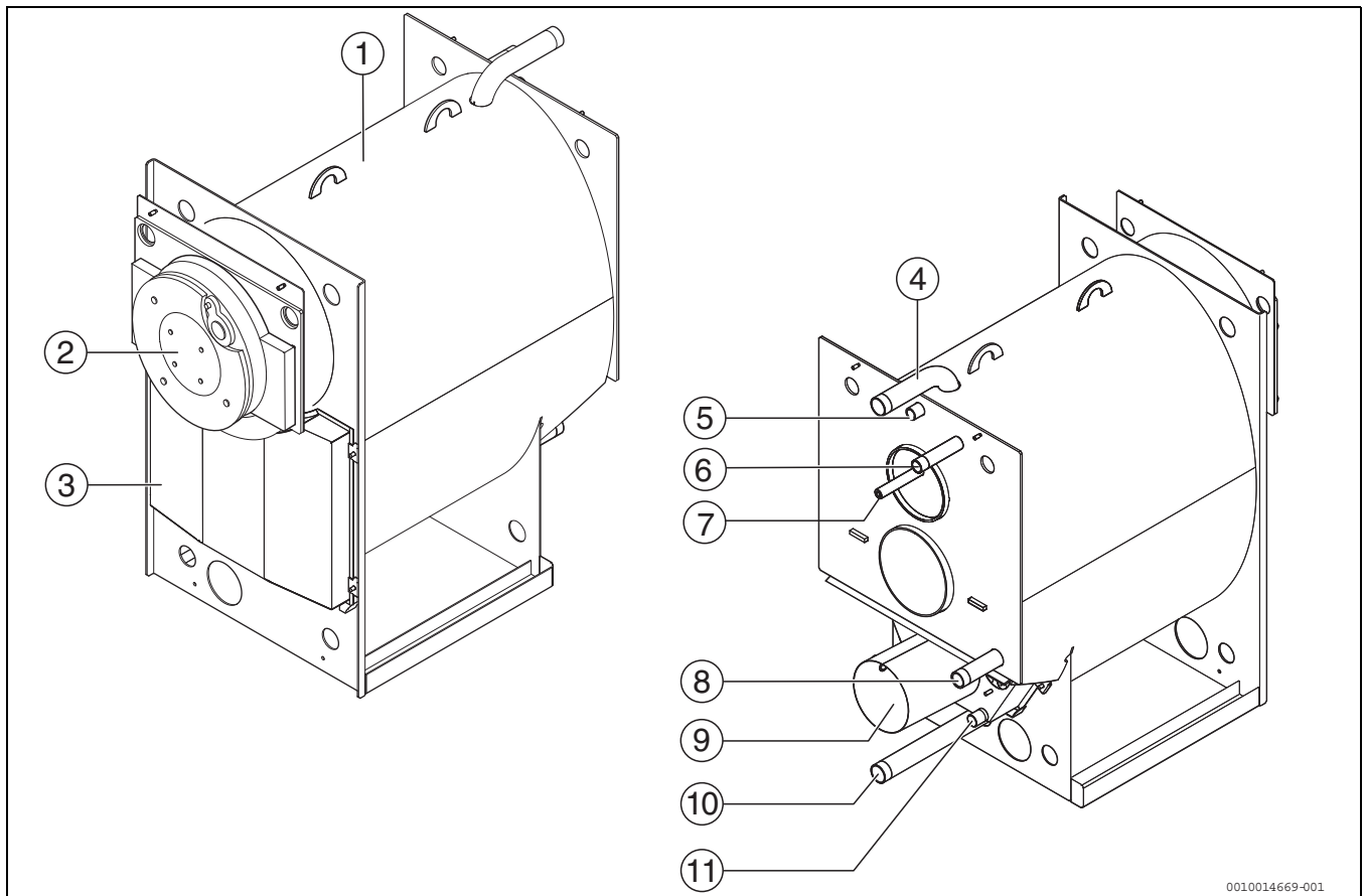
Bild 2 Kesselübersicht
