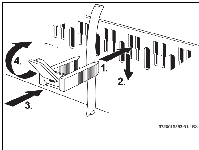
Bild 34 Kabel mit Kabelschelle sichern
