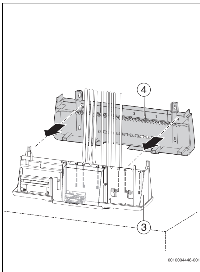
Bild 35 Montage auf Kessel, aufstecken Rückwand einrasten
