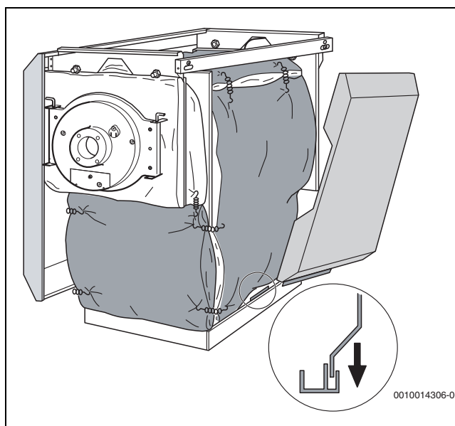
Bild 18 Seitenwände einsetzen
