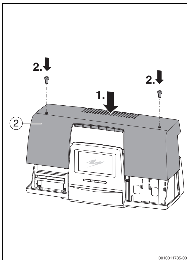
Bild 40 Abdeckhaube am Regelgerät montieren
