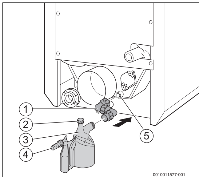
Bild 13 Kondensatleitung installieren
