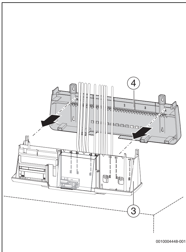
Bild 37 Rückwand am Gehäuseunterteil befestigen
