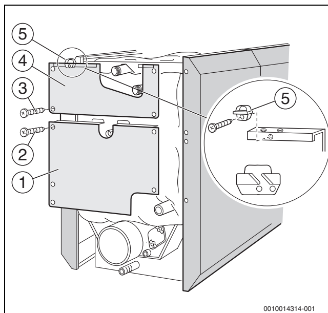
Bild 20 2-teilige Rückwand anschrauben
