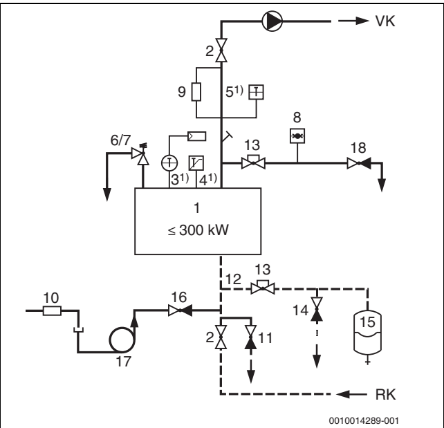
Bild 46 Sicherheitstechnische Ausrüstung nach EN 12828:2012 für Kessel ≤ 300 kW mit Sicherheitstemperaturbegrenzer (STB) ≤ 110 °C
