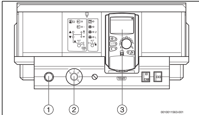
Bild 32 Einstellungen am Regelgerät
