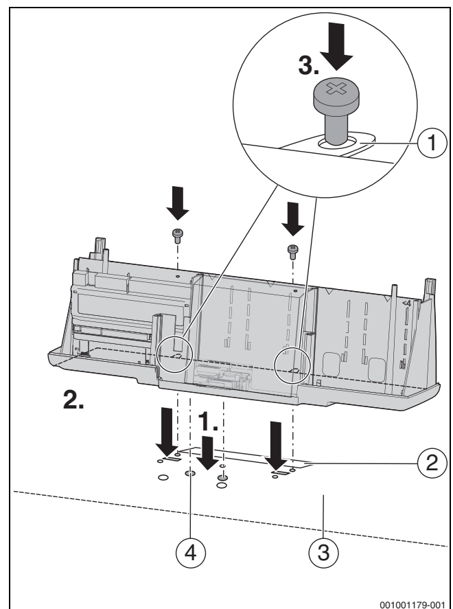
Bild 33 Regelgerät montieren
