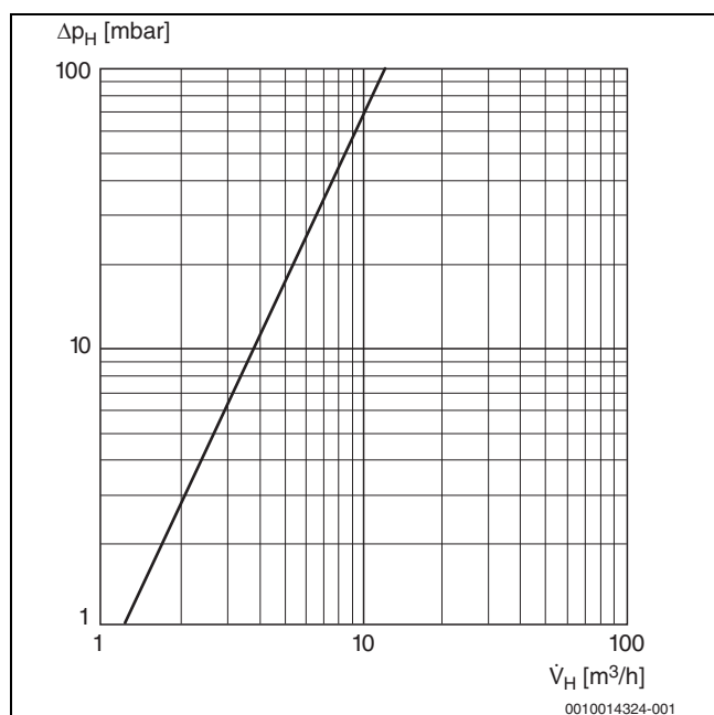
Bild 47 Wasserseitiger Durchflusswiderstand
