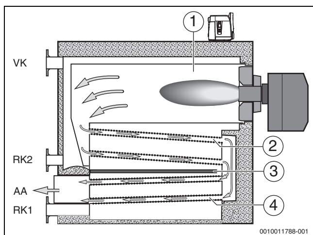
Bild 1 Funktionsschema des Heizgasverlaufs beim Brennwertkessel Logano plus SB325
