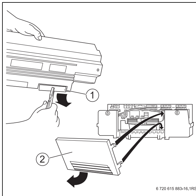
Bild 30 Kabeldurchgang vorbereiten
