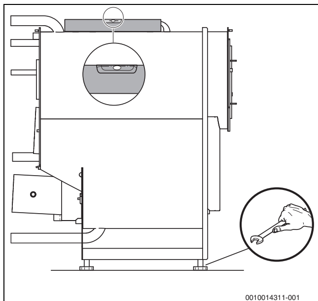
Bild 8 Kessel ausrichten
