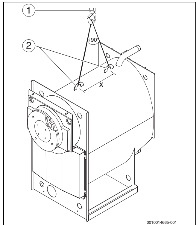
Bild 4 Kessel mit einem Kran heben
