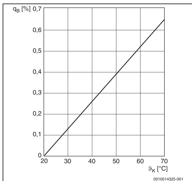
Bild 48 Betriebsbereitschaftsverlust in Abhängigkeit von der mittleren Kesselwassertemperatur
