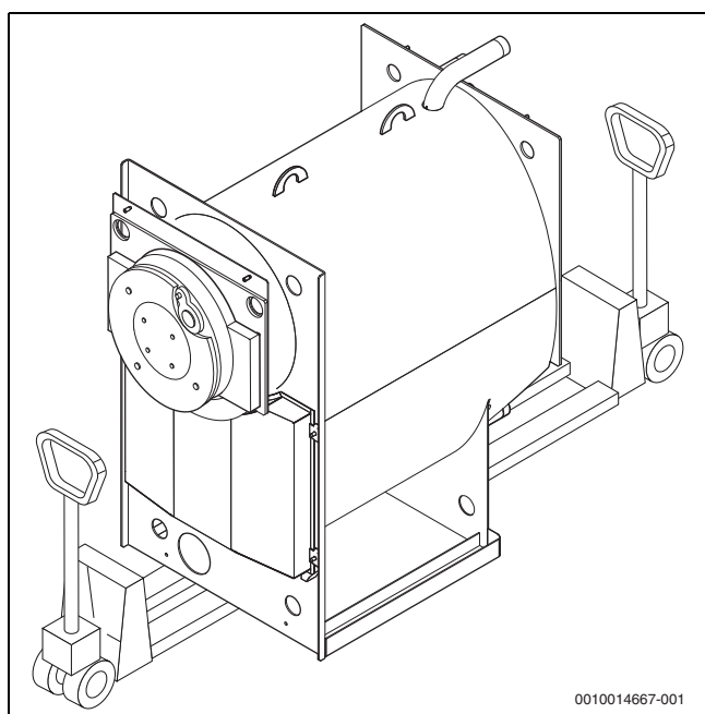
Bild 6 Kessel mit 2 Hubwagen transportieren
