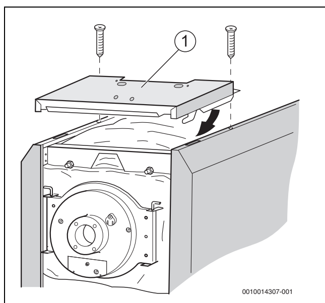
Bild 21 Vordere Kesselhaube montieren
