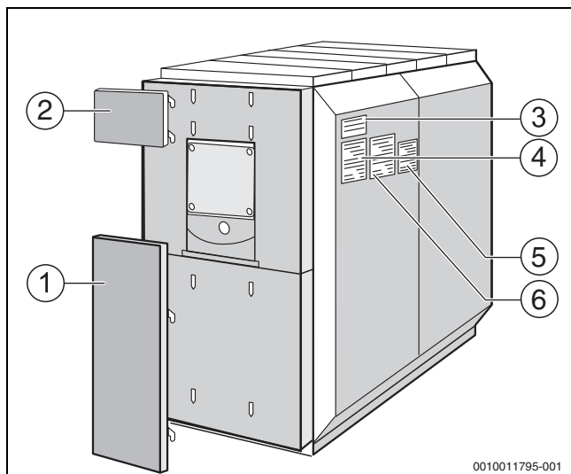
Bild 26 Typschild befestigen
