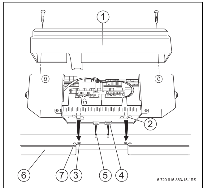
Bild 29 Regelgerät montieren
