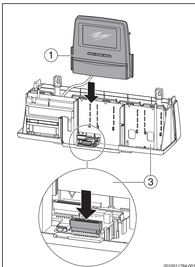
Bild 39 Bedieneinheit am Gehäuseunterteil einstecken
