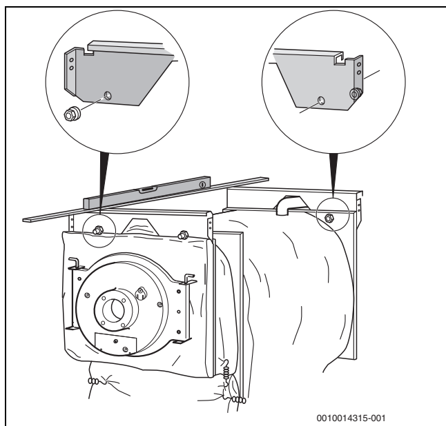
Bild 16 Vordere und hintere Traverse einsetzen und verschrauben
