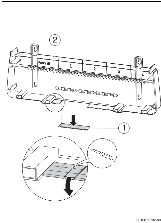
Bild 36 Kabeldurchgang vorbereiten
