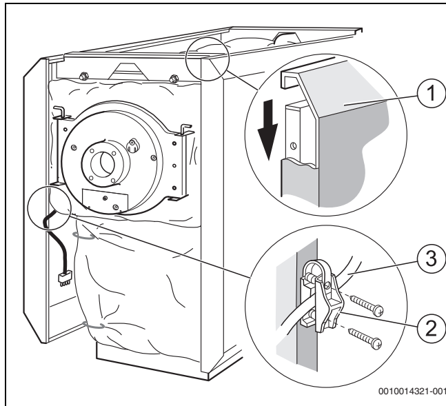
Bild 19 Seitenwände einhängen und Brennerkabel anbringen
