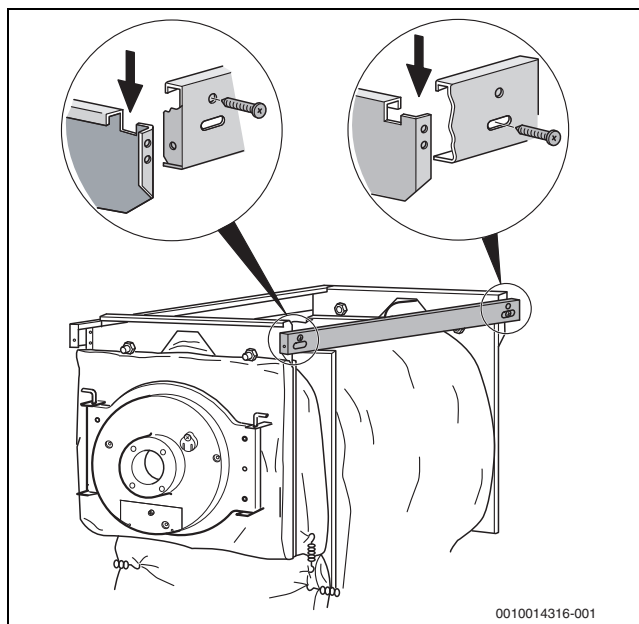
Bild 17 Seitliche Traversen einhängen und anschrauben
