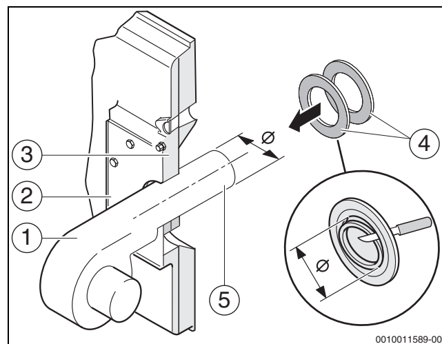
Bild 25 Brenner montieren
