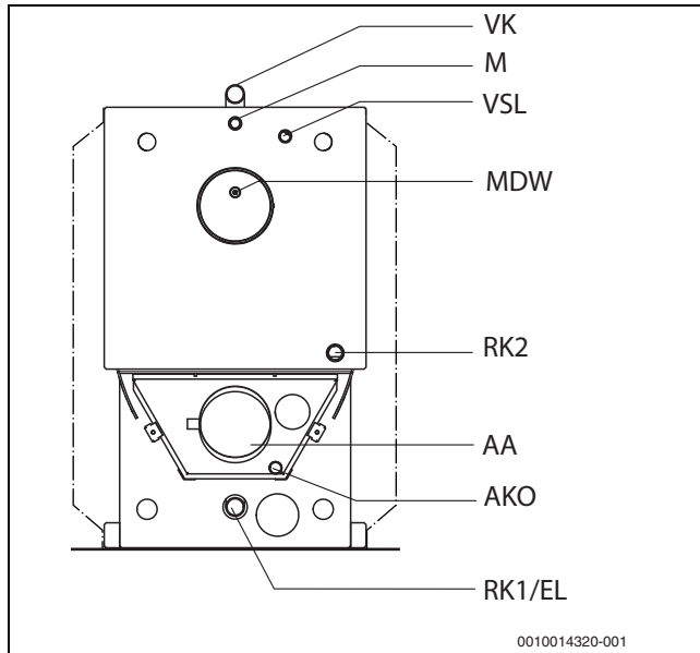
Bild 15 Anschlüsse am Kessel Logano plus SB325
