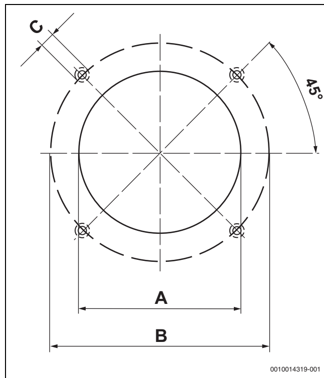
Bild 24 Brenneranbaumaße in Feuerraumtür
