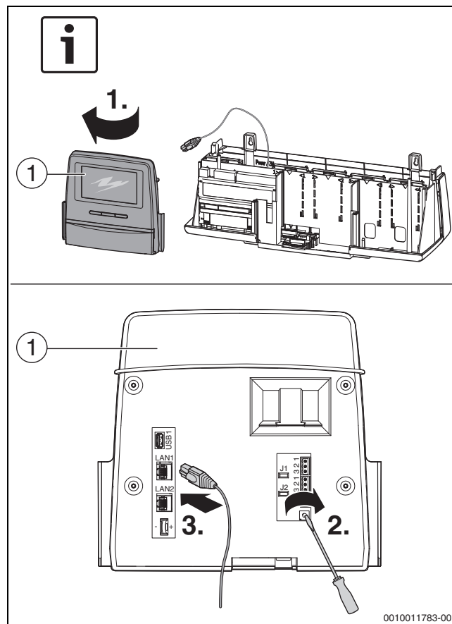
Bild 38 Regelgeräteadresse einstellen
