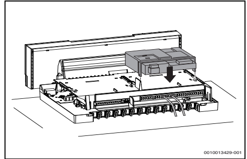
Bild 6 Fremdbrennermodul einsetzen und einrasten lassen
