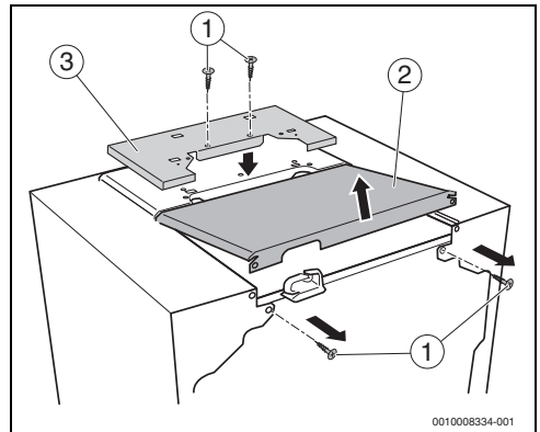
Bild 7 Hintere Kesselhaube abnehmen/Adapterblech montieren
