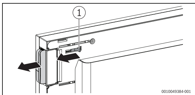
Bild 5 Kommunikationsmodul demontieren
